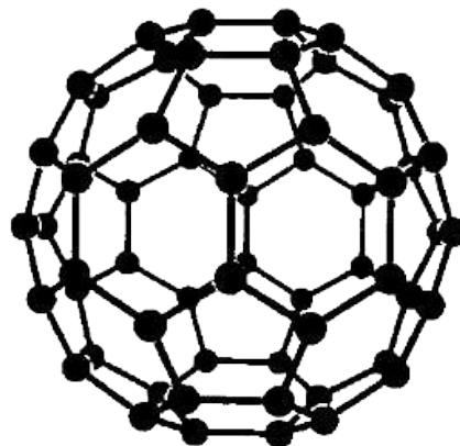
C60
